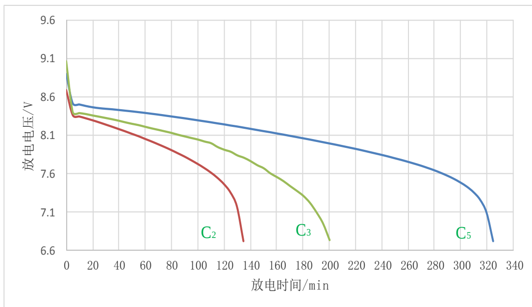
电池 C 2 、C 3 、C 5 容量的放电曲线
